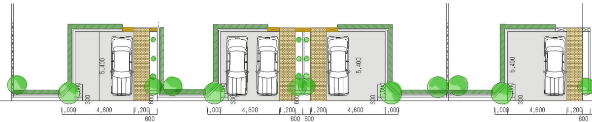
並列駐車
